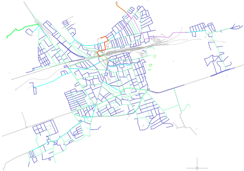
რუკა 1. საშურის წყლის გამანაწილებელი საპროექტო სისტემა
